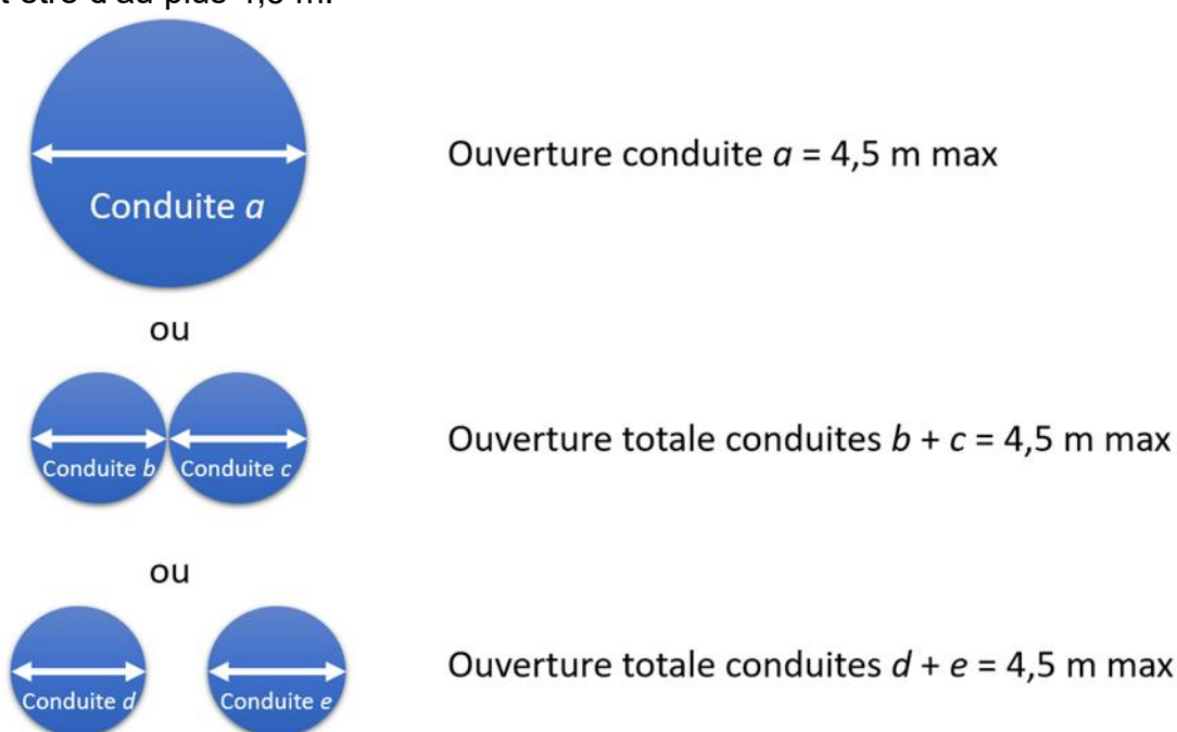
Figure 327.1 : Croquis illustrant l'ouverture permise d'un ponceau selon le nombre de conduits
